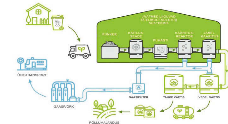
Tehase skeem
